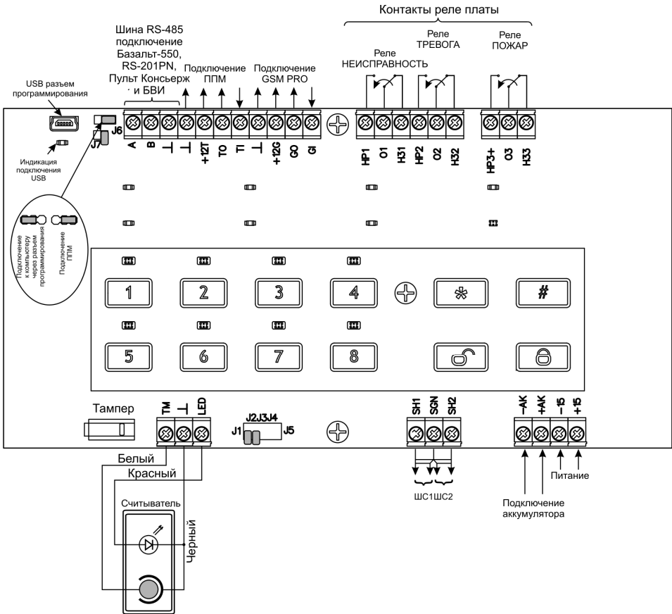
Рисунок 11 – Монтажная схема платы охранной панели ретранслятора
