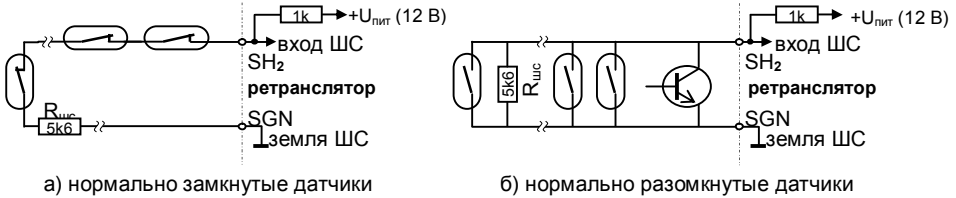
Рисунок 9 – Примеры монтажа охранных шлейфов
