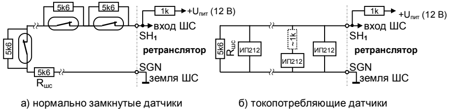
Рисунок 10 – Примеры монтажа пожарных шлейфов
